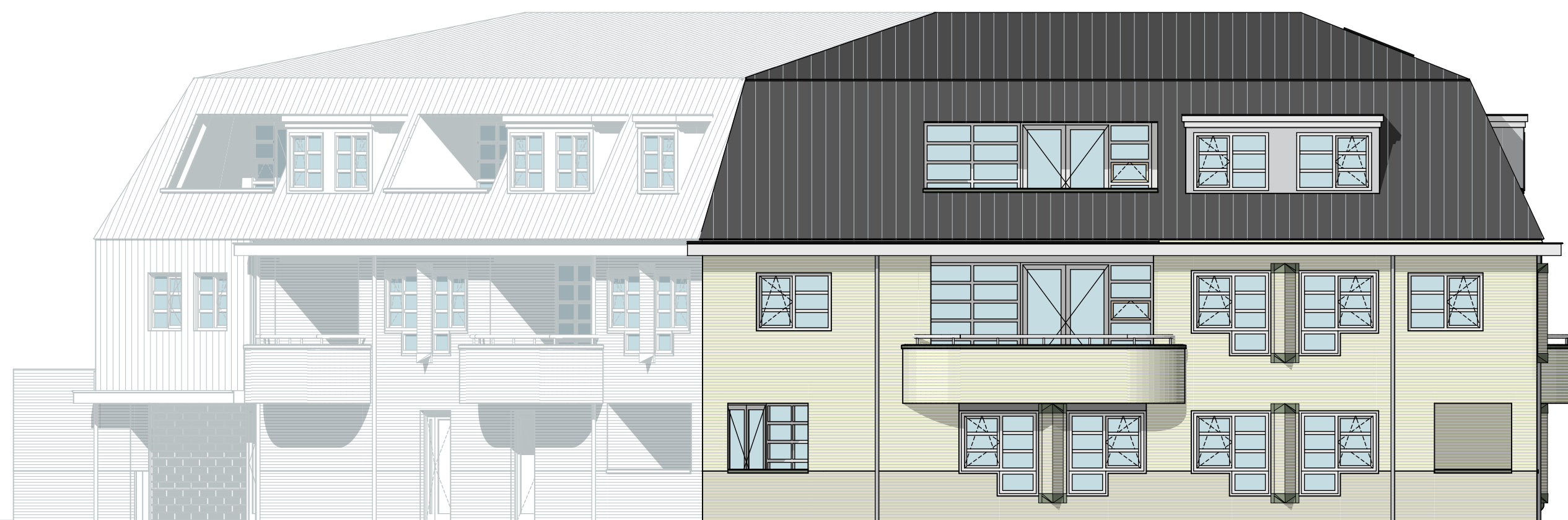
LINKERZIJGEVEL
