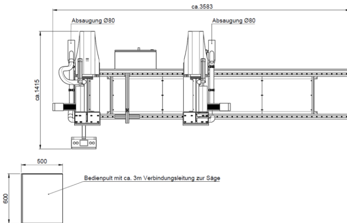
Bovenaanzicht Exenso DS350 3.000 mm - Technische wijzigingen voorbehouden
